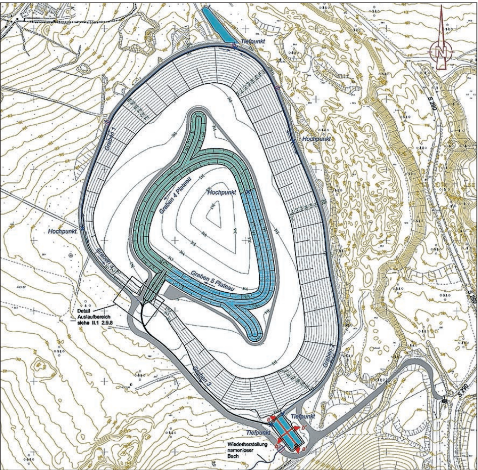
LAGEPLAN MIT DARSTELLUNG DER KONTUREN UND DES WASSER- UND WEGEBAUS IM ENDZUSTAND. ABBILDUNG: WISMUT GMBH
