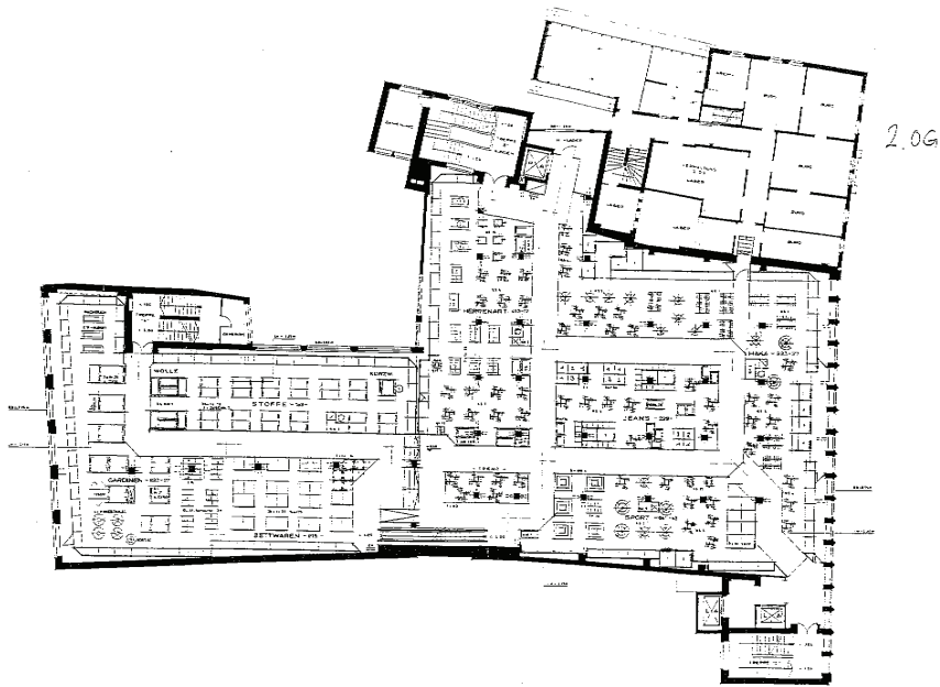
Grundriss 2. OG, ca. 1955
